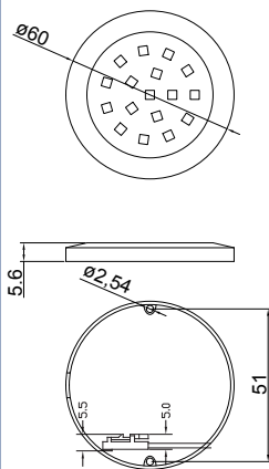
Размеры светильника
